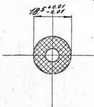
Sezione AB
