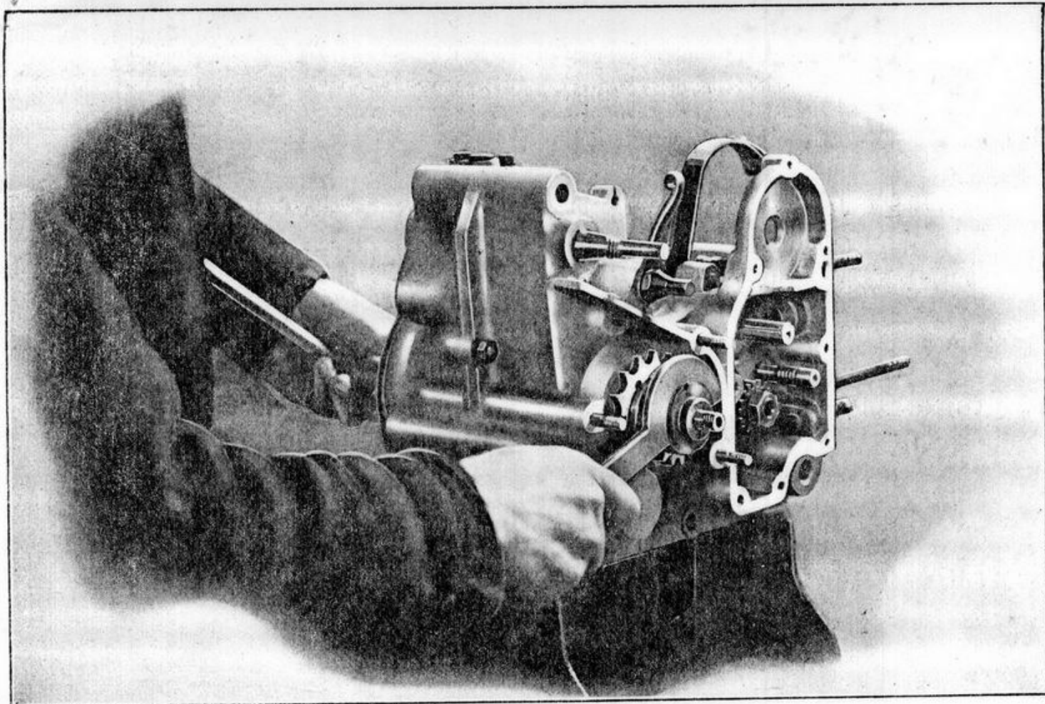
Fig. 16 - Come si leva il manicotto dentato per la messa in moto
