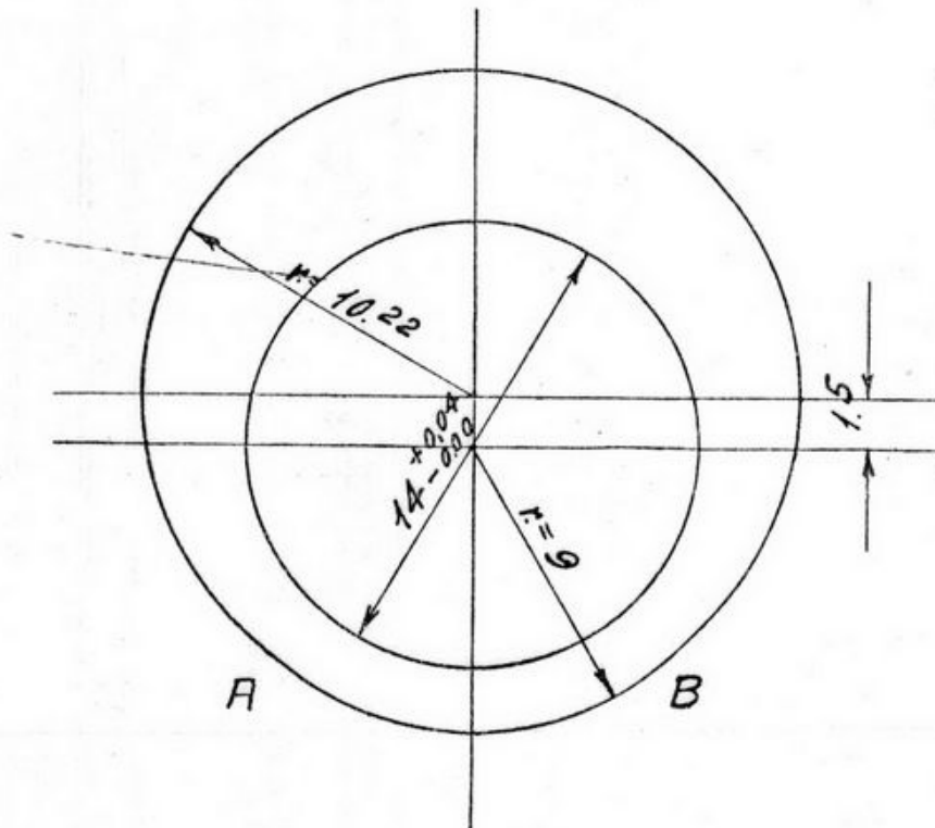
Fig. 29 - Schema sede delle palette della pompa ricupero
