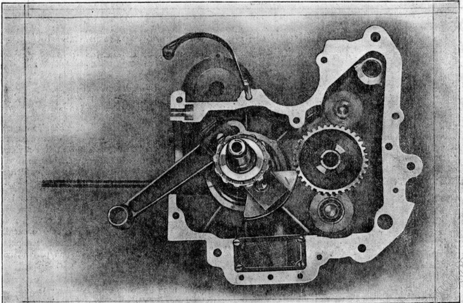
Fig. 20 - Ecco il mezzo carter destro così come si trova appena operata la separazione. Si notino montati l'albero a gomito completo e l'ingranaggio per presa diretta del cambio.
