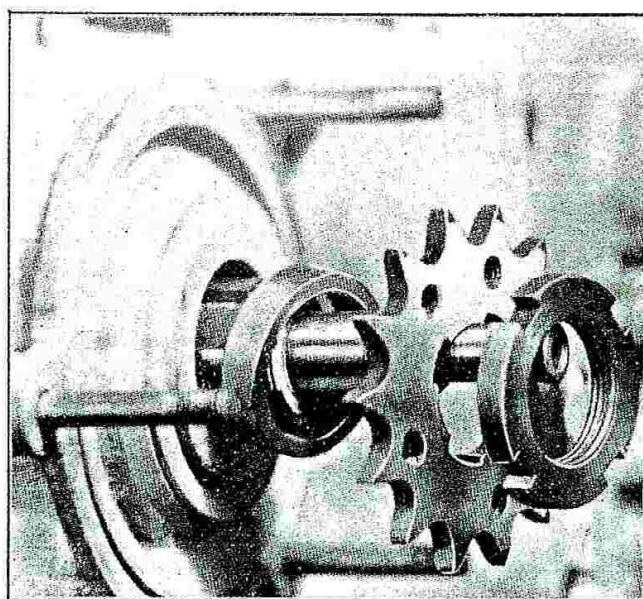
Fig. 45 - Come, dopo allentata la ghiera di serraggio, si levano il pignone e l'anello spessore.
