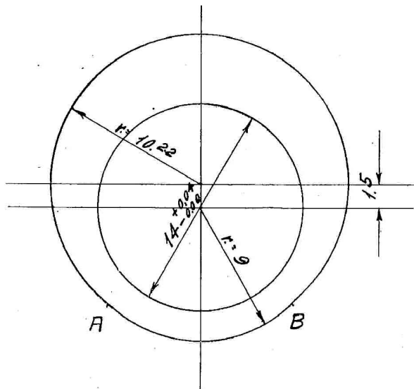
Fig. 73 - Schema sede delle palette.
