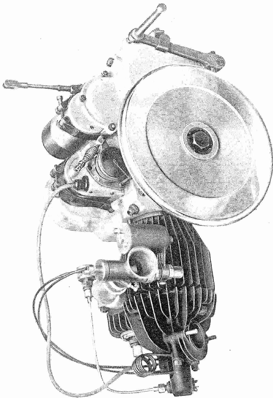
Fig. 2 - Gruppo motore cambio, lato volano
